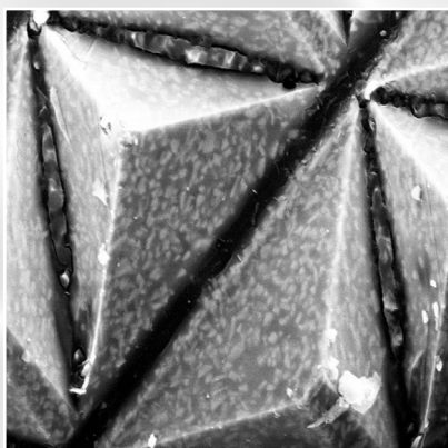
Уникальный абразив Trizact имеет форму пирамиды (50079)
