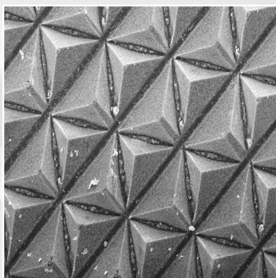
Упорядоченное строение абразивных пирамид Trizact
